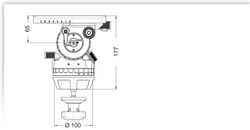
Abmessungen
