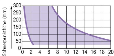
Kameraplattform Gewichtsausgleich
